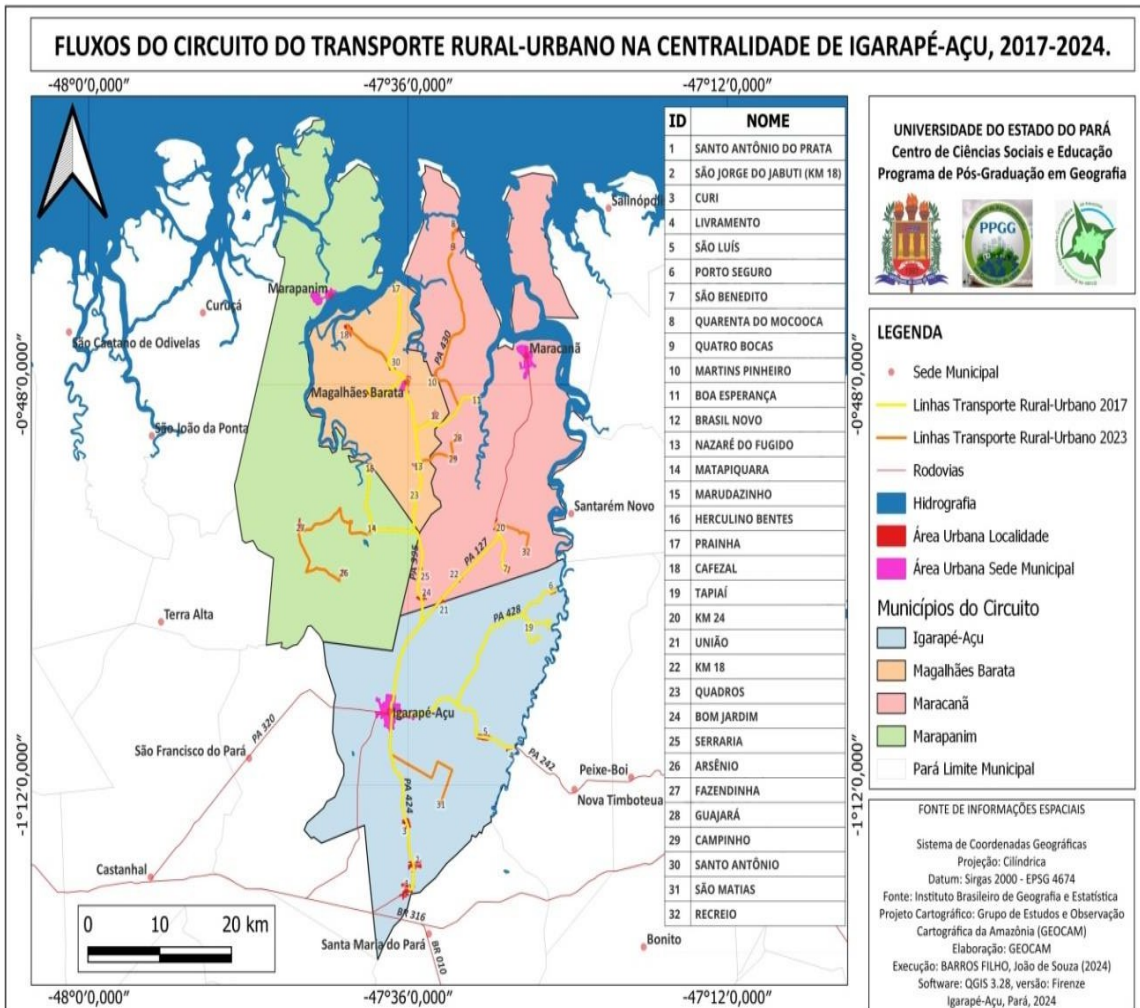
Mapa 1: Dinamismo espacial do transporte rural-urbano na nova centralidade econômica de Igarapé-Açu, 2017-2024.
