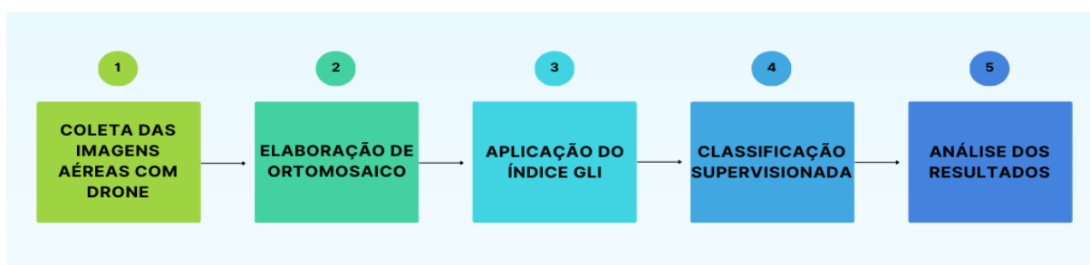
Figura 3. Fluxograma do processo de obtenção dos dados geoespaciais.
