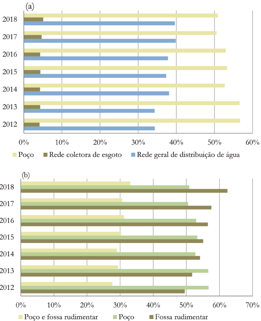
Gráfico 1 - Representação gráfica da condição de acesso ao saneamento básico pelas pessoas inscritas no Cadastro Único - região de Carajás, 2012-2018.
