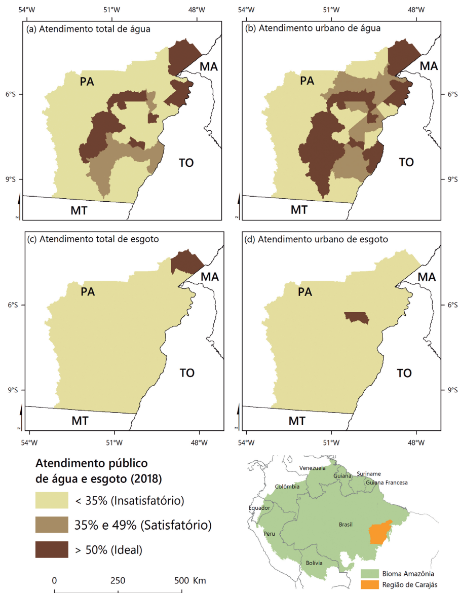
Figura 5 - Mapas com representação de diagnóstico geral das condições de saneamento da população da região de Carajás inscrita no Cadastro Único no ano de 2018.
